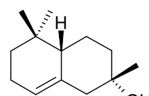
alpha-ambrinol
